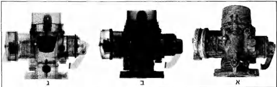
א. קרדורטר של סגנונית; ב. כפי שצולם בקרינה X; ג. כפי שצולם בניטרונים
